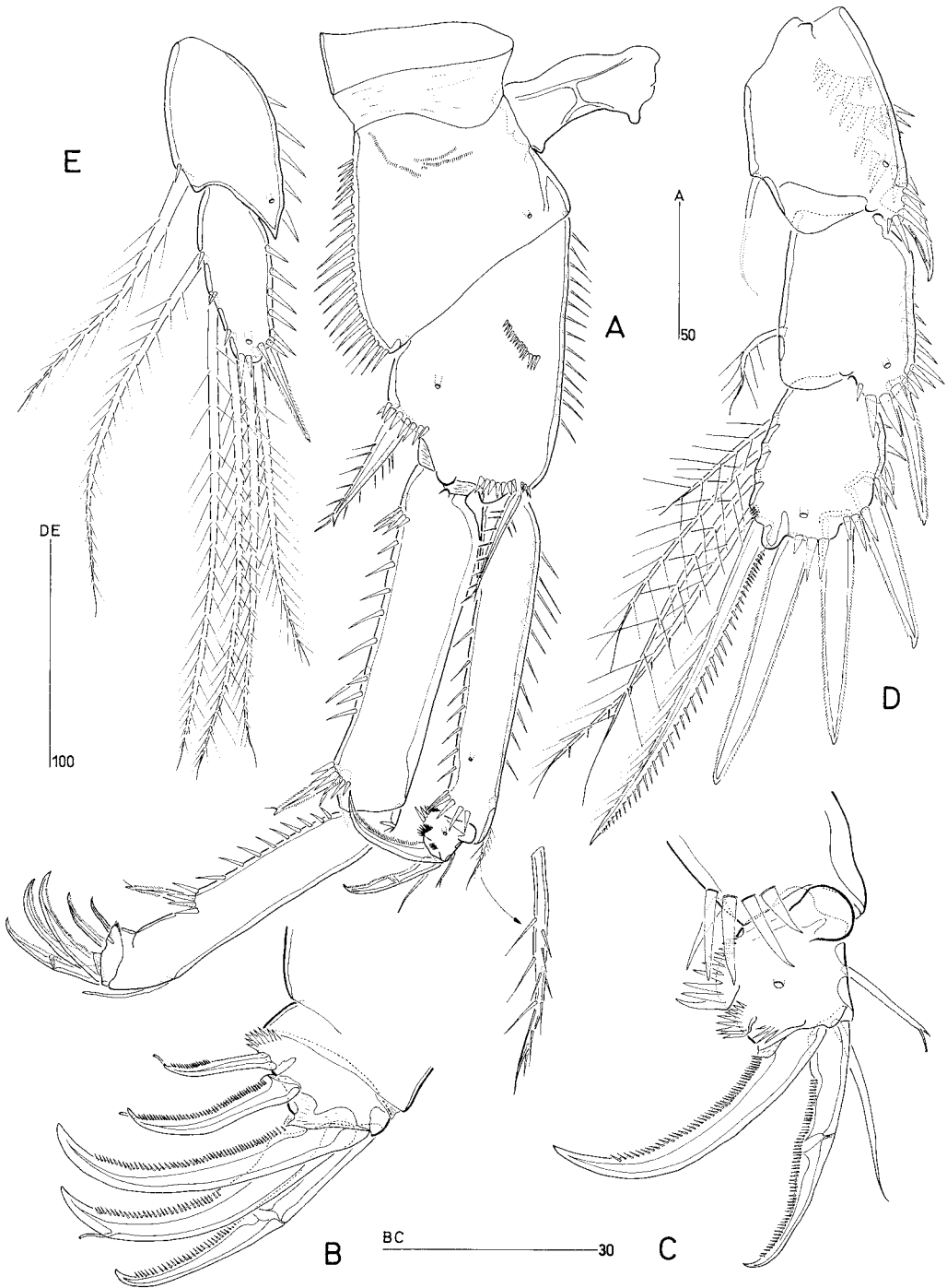
Fig. 5. Harpacticus spartacus (Leigh-Sharp, 1936), new combination (♂). A, P1, anterior [insert showing inner seta of enp-1]; B, P1 exp-3, anterior; C, P1 enp-2, anterior; D, P3 exopod, anterior; E, P3 enp-2 and -3, anterior.
