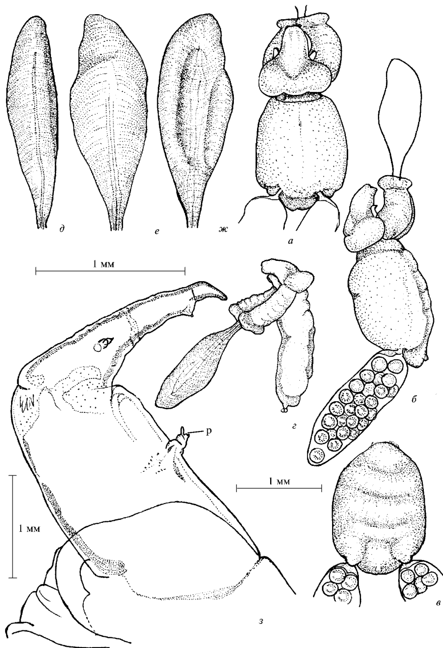
Рис. 1. Salmincola mica , ♀: а — половозрелая самка, общий вид, дорсально; б — то же, латерально; в — то же, вентрально; з — молодая взрослая самка, латерально; д-ж — булла; з — максиллепада, общий вид (р — сосок).
